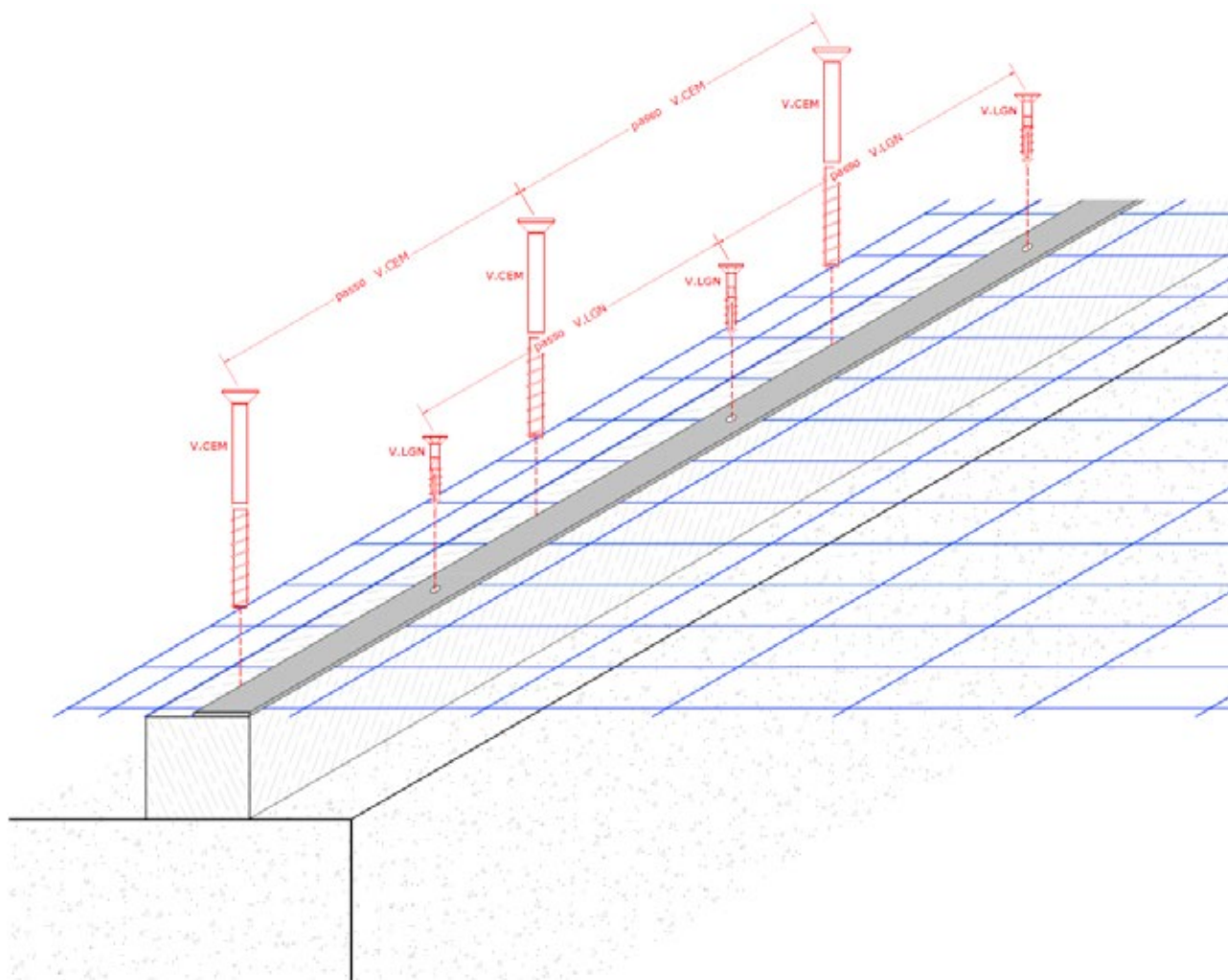
Figura 1 - Schema individuazione passo Fissaggi
