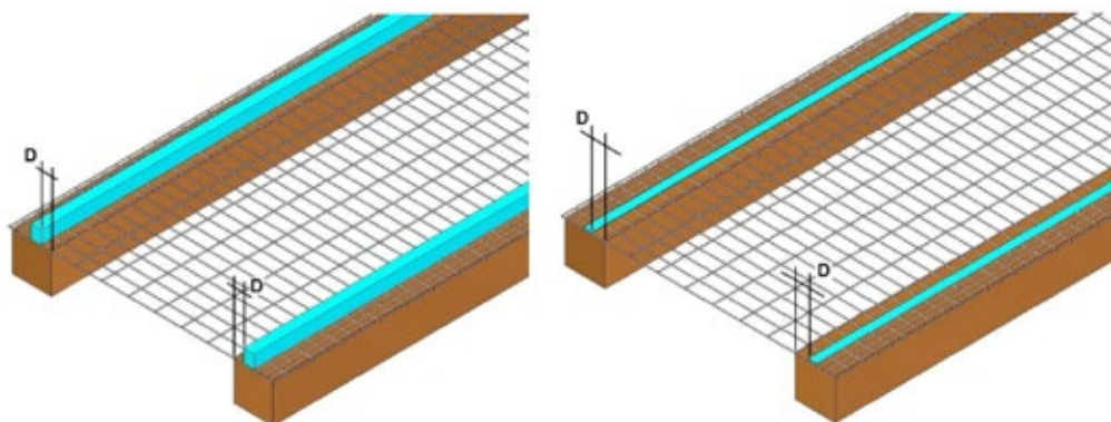
Figura 17 – Distanza dal bordo degli elementi di fissaggio
