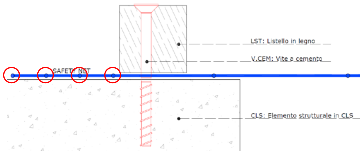
Figura 12 – Modalità installazione rete
