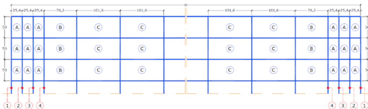
Figura 11 – Schema dimensionale delle maglie della rete SAFETY NET
