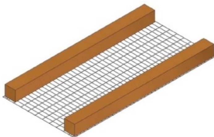
Figura 9 – Installazione DOWN: rete in posizione inferiore rispetto al Supporto principale
