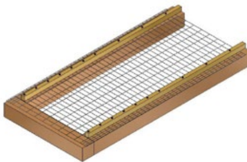
Figura 16 – Chiusura senza elemento di Supporto
