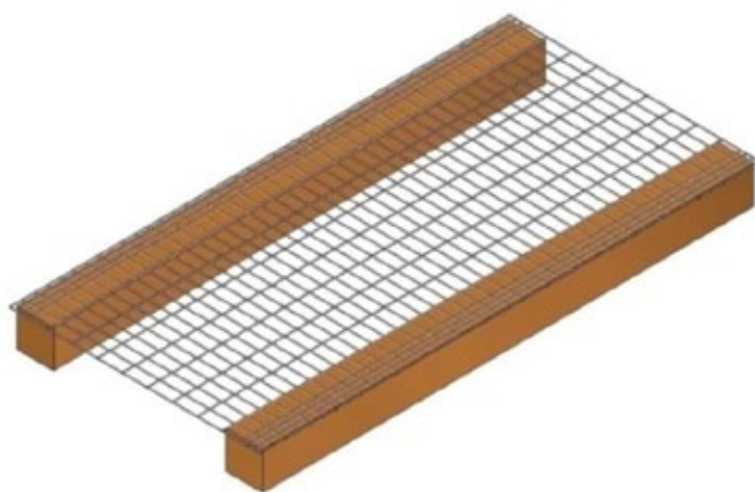
Figura 8 – Installazione UP: rete in posizione superiore rispetto al Supporto principale
