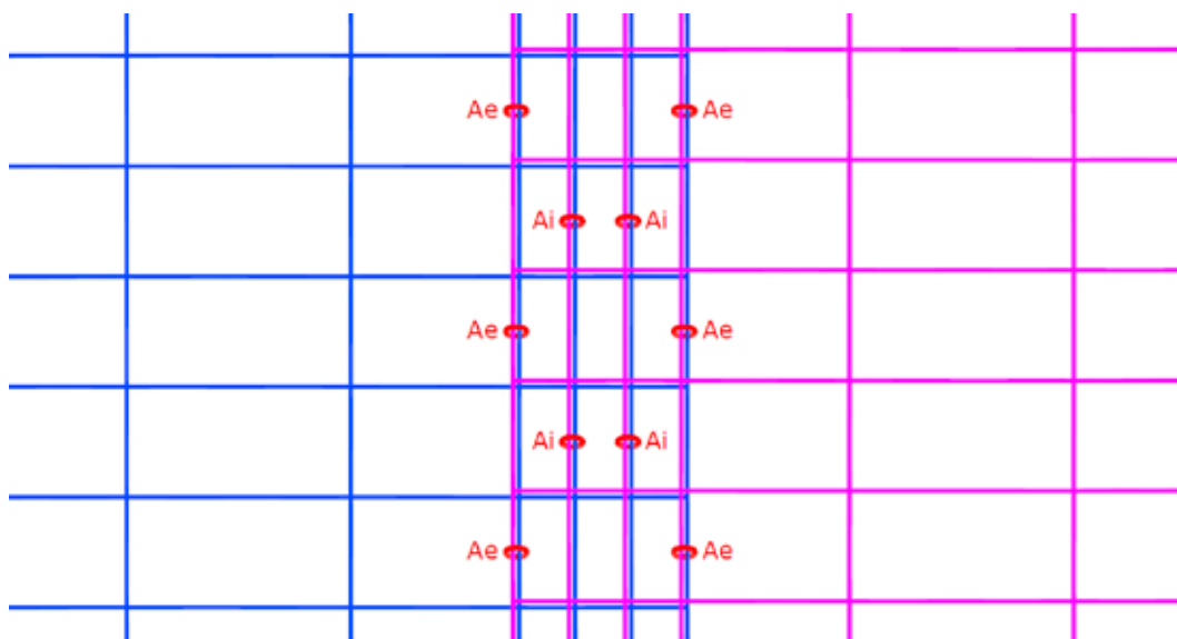
Figura 14 - Schema di Giunzione Longitudinale con Anellature tra 2 rotoli adiacenti di rete
