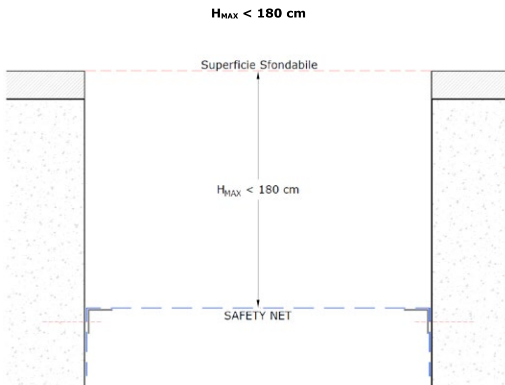
Figura 10 - Distanza massima di installazione da superficie sfondabile
