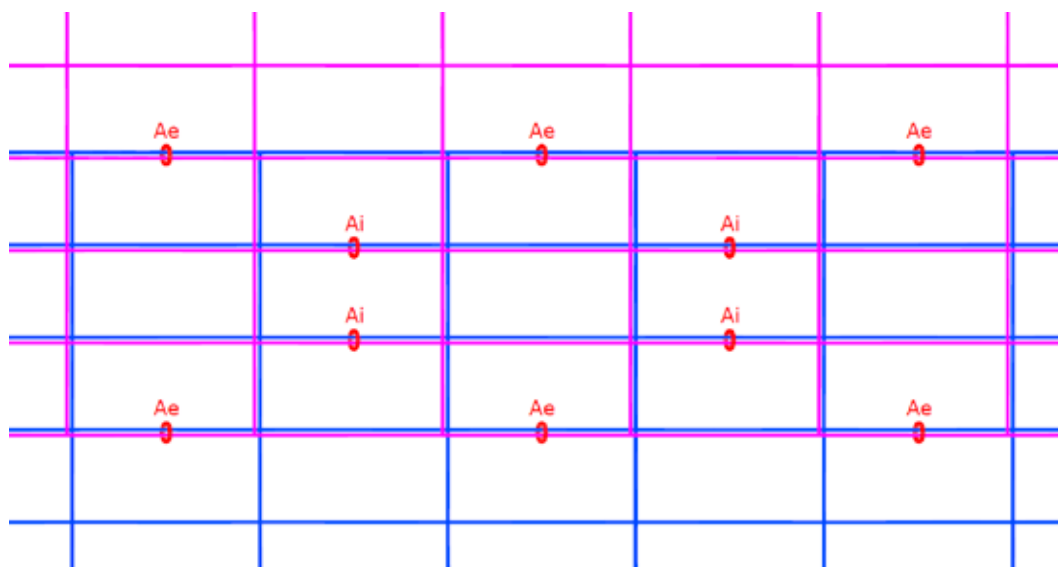
Figura 13 – Schema di Giunzione Trasversale con Anellature tra 2 rotoli consecutivi di rete
