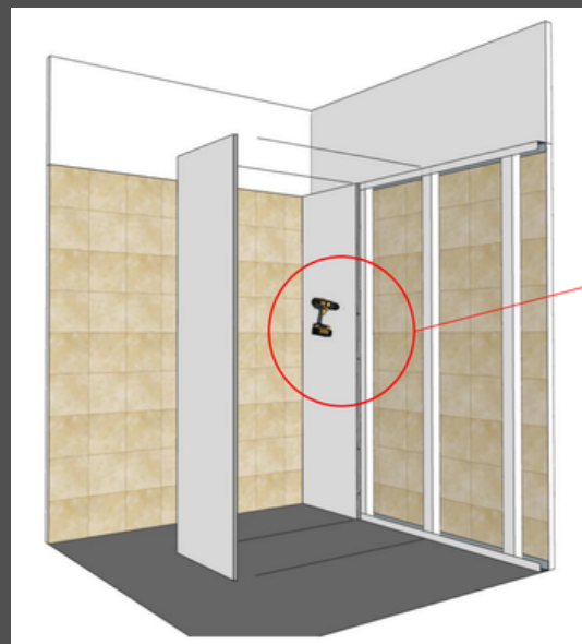
Fig. 3 - Fissaggio pannelli su struttura di supporto
